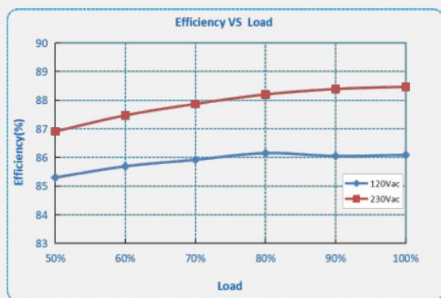
F1-060X-054 ( I_o=1.4A )
